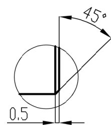
DETALLE H ESCALA 2 : 1
